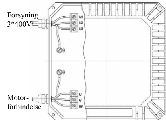
Fig. 5 Monteringsoversigt for HV 3.15 og 2.23
