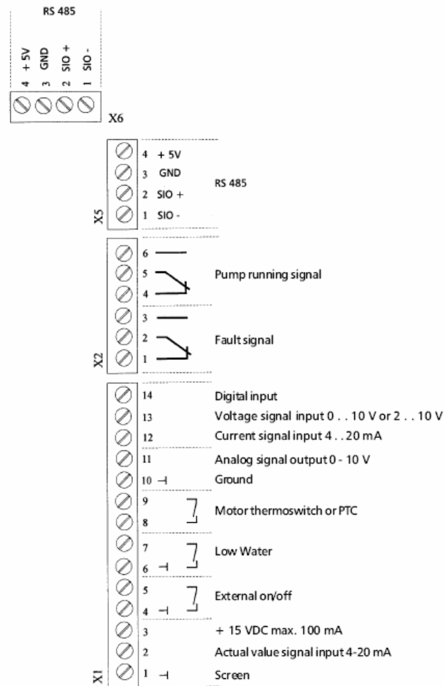
Fig. 7 Tilslutningsoversigt
