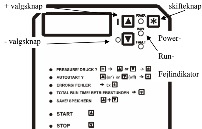
Fig. 3 Betjeningspanel
