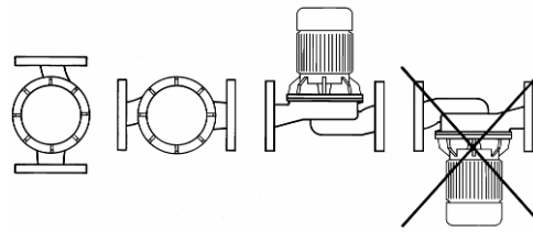
Fig. 1 Pumpeorientering
