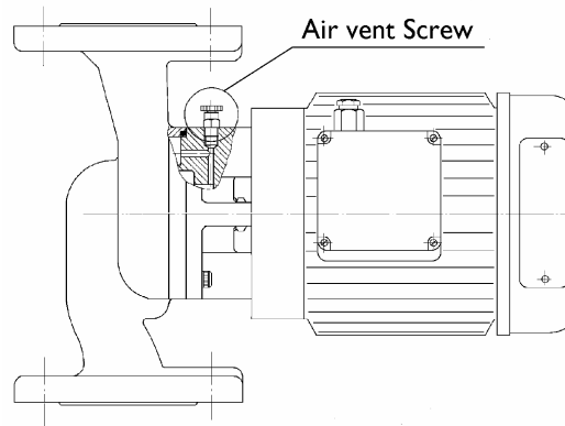
Fig. 2 Udluftningsskruens placering
