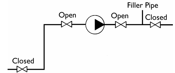
Fig. 4 Placering af pumpe og afspærringsventiler
